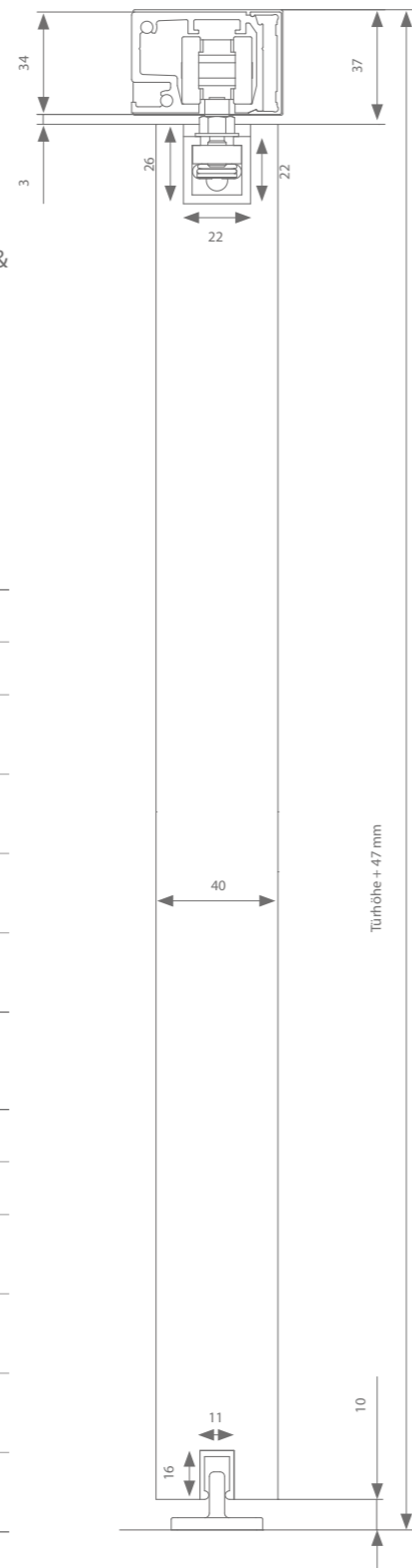
Technische Zeichnung
