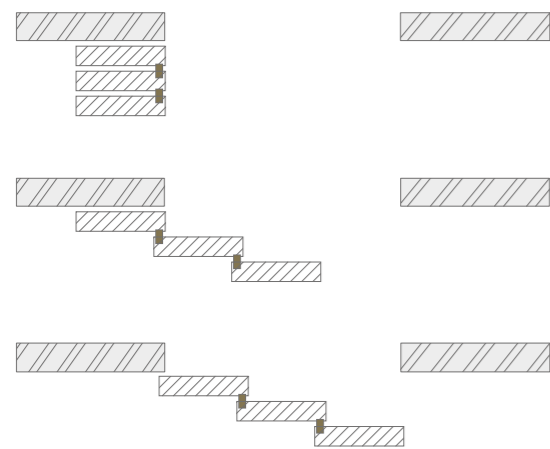
Version mit Mitnehmern
