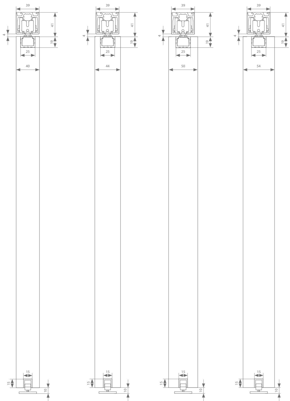
Deckenmontage 40 mm Deckenmontage 44 mm Deckenmontage 50 mm Deckenmontage 54 mm
