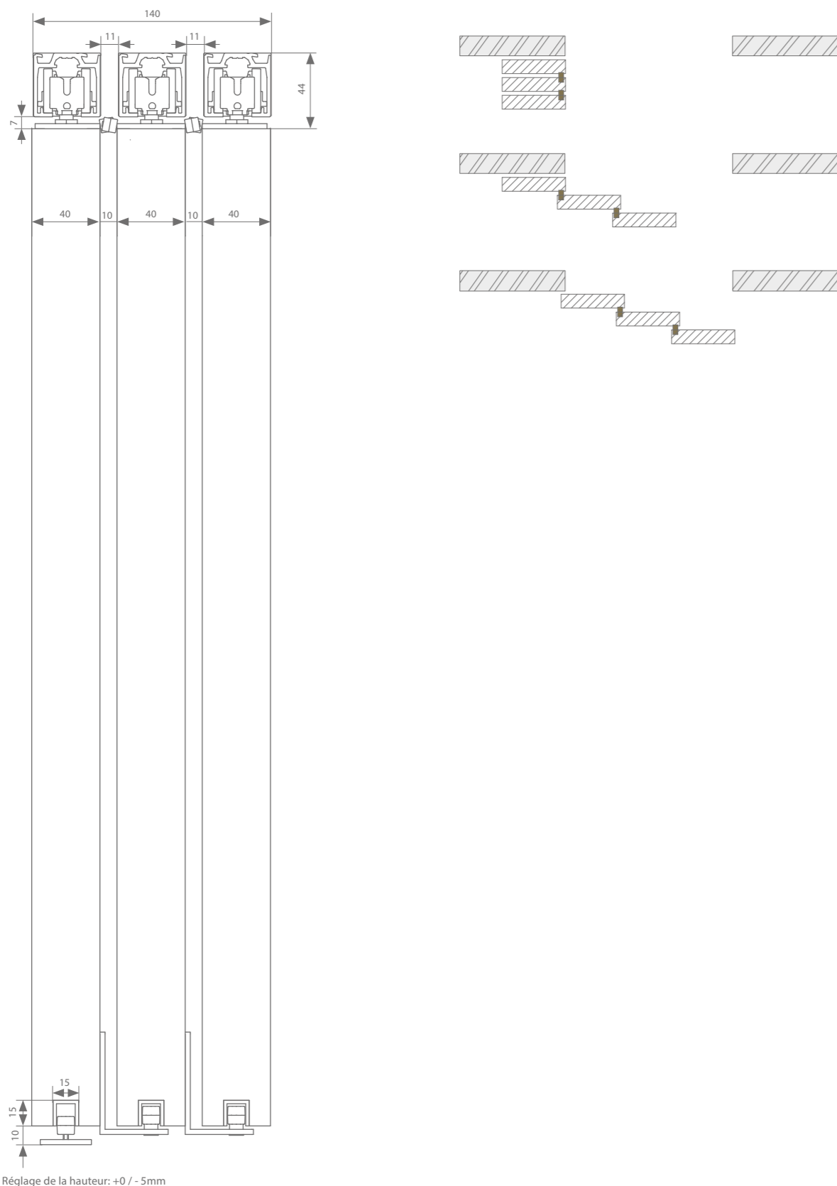
Réglage de la hauteur: +0 / - 5mm
