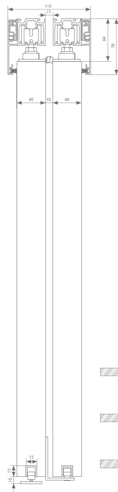
fixation parallèle au plafond 2
